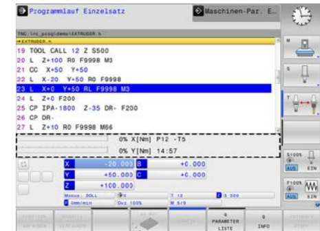
Kleines PLC-Fenster
